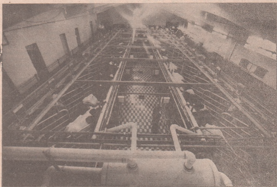
МОСКОВСКАЯ ОБЛАСТЬ. В Подольском районе в агрофирме «Шапова» работает новейшая доильная установка (на снимке), не имеющая аналогов в СССР и Европе. Она изготовлена по совместному проекту СССР и США американской фирмой «Бабсон Бразерс».
